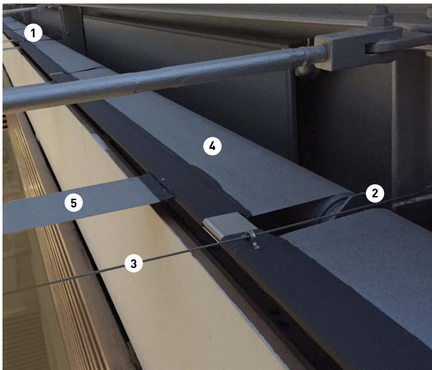
Ill.: JM-Horizontal FTS, frithængende dug med trækbændel
